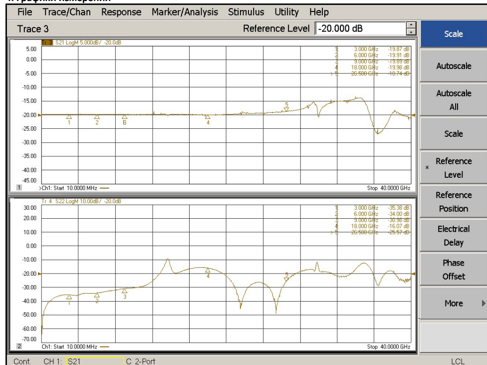
Графики для АЧХ при отсчётном уровне равном -20 дБ
